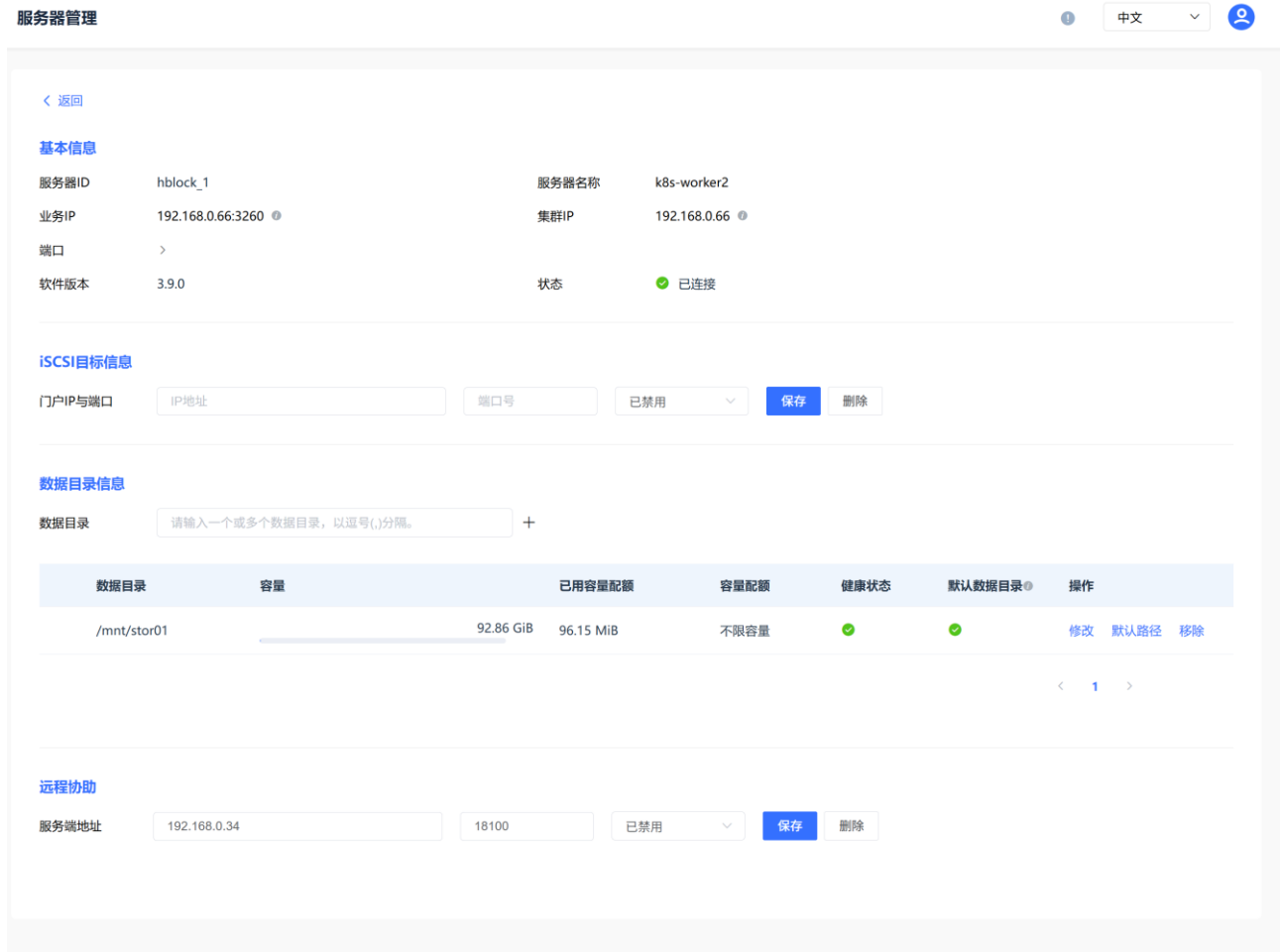
图79. 服务器详细信息（单机版）
