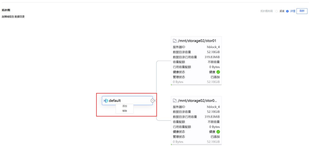
图55. 为已有节点的存储池添加节点
