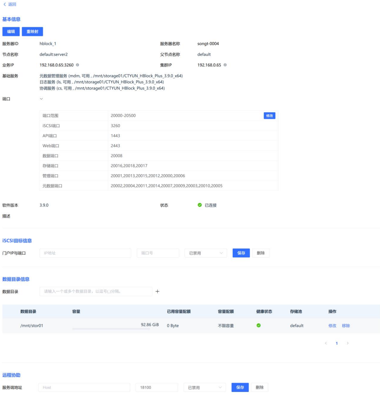
图80. 服务器详细信息（集群版）
