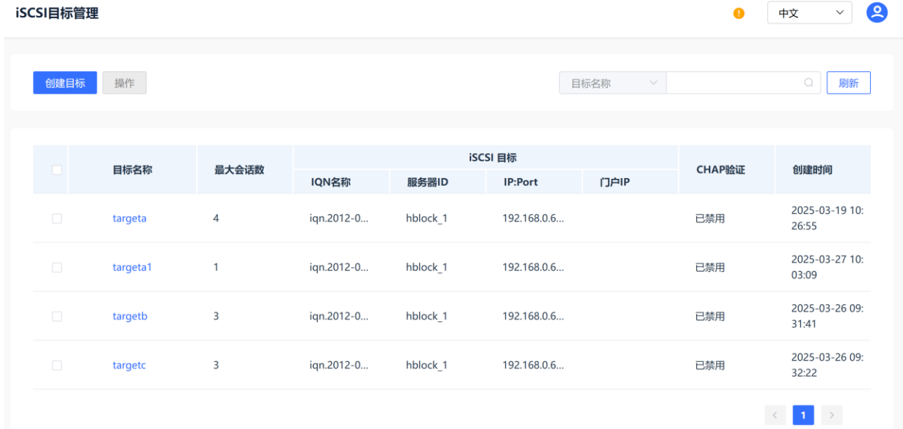
图43. iSCSI 目标管理（单机版）
